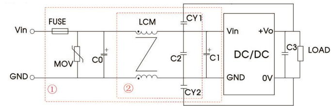
图 4 注：图 4 中第①部分用于 EMC 测试；第②部分用于 EMI 滤波，可依据需求选择。
